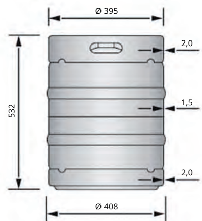
bokorys sud KEG 50 l
