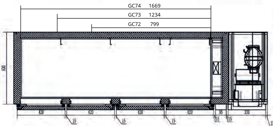
Přední strana GC
